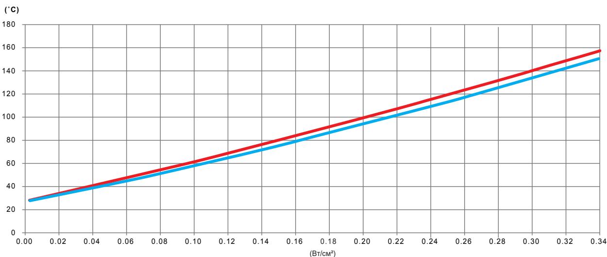
Изменение в зависимости от мощности в Вт/см 2 силиконовой нагревательной ленты и температуры стенки пустой нержавеющей стальной трубы, теплоизолированной 20 мм пеной PVC-NBR
