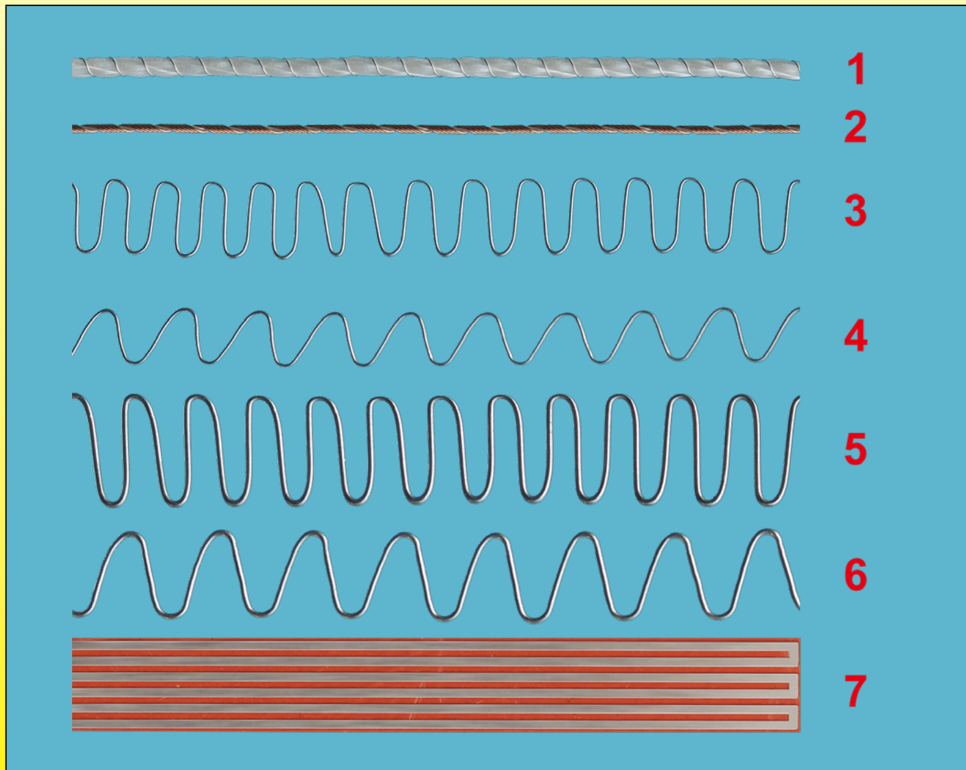
1: Намотка вокруг стекловолоконного сердечника с 1-6 параллельно расположенными проводниками; 2: Намотка вокруг арамидного сердечника с 1-6 параллельно расположенными проводниками; 3, 4, 5, 6: Плоская зигзагообразная пружина; 7: Нагревательная сетка, изготовленная методом химического травления металлической фольги.
